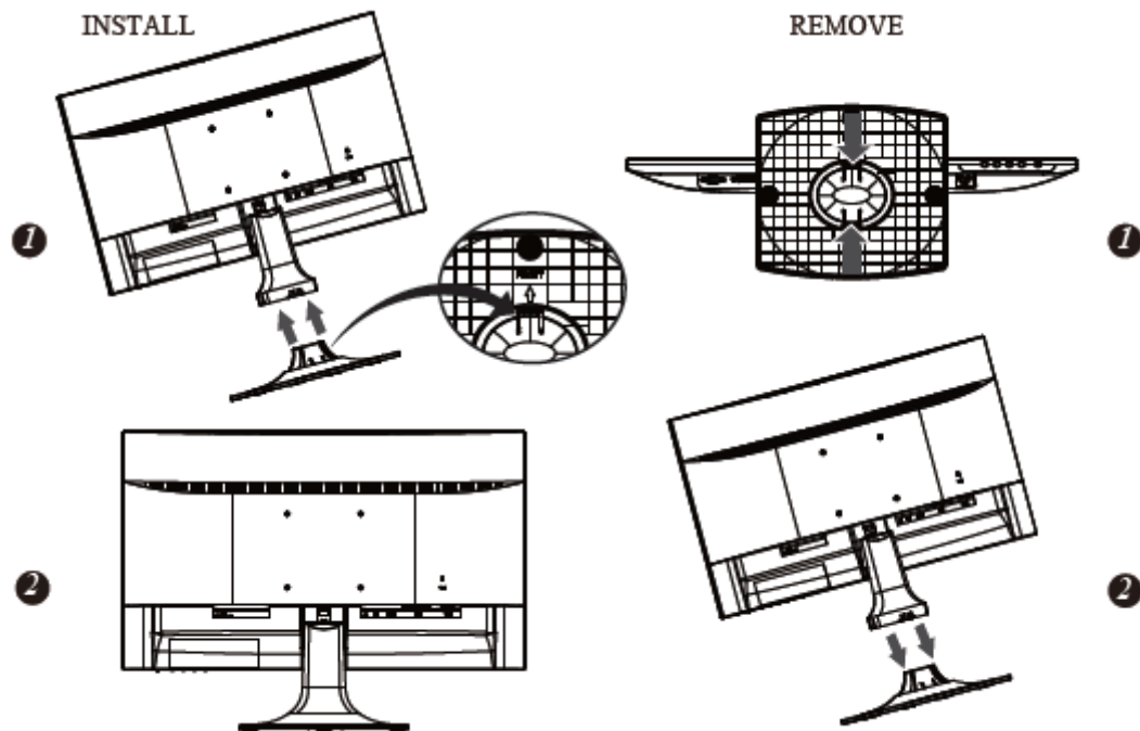
Figura.1. Installazione e Rimozione della Base
