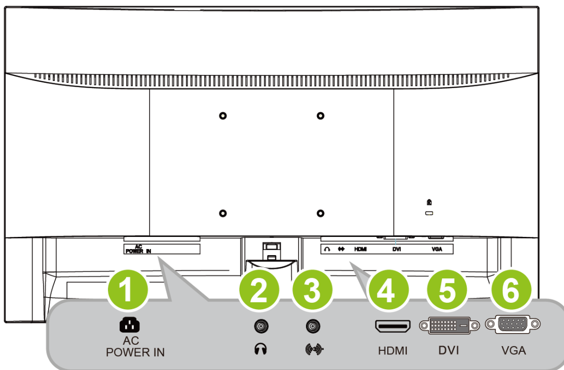
Figura 2. Collegamento al pc
